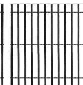
Radius Z10155 Slot 15,5mm Open area 76,5%
